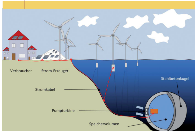
ABB. 1 | MEERES-DRUCKSPEICHERKRAFTWERK
